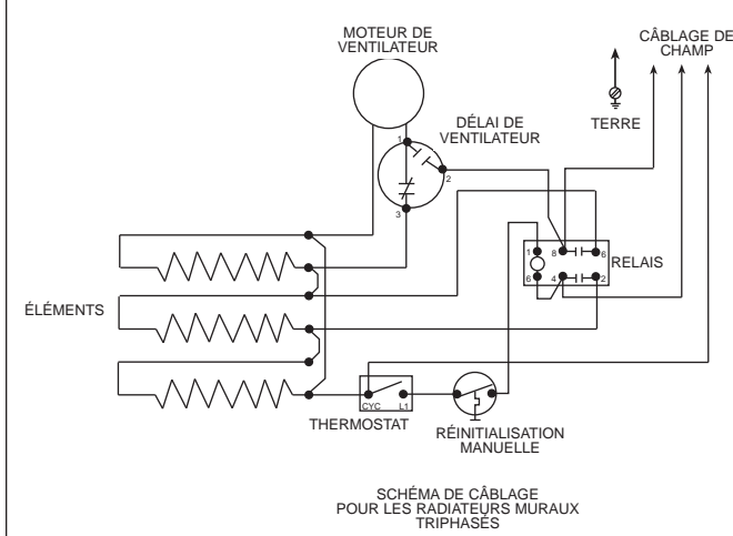
Fig. 5 Schémas de câblage
